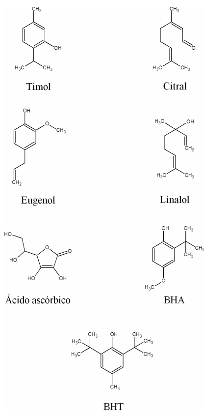
Figura 1 – Estruturas químicas do timol, citral, eugenol, linalol, ácido ascórbico, BHA E BHT
